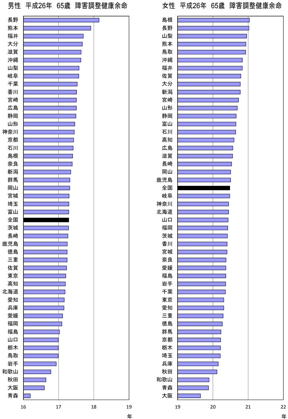
平成26年 47都道府県 65歳 障害調整健康余命(DALE)
