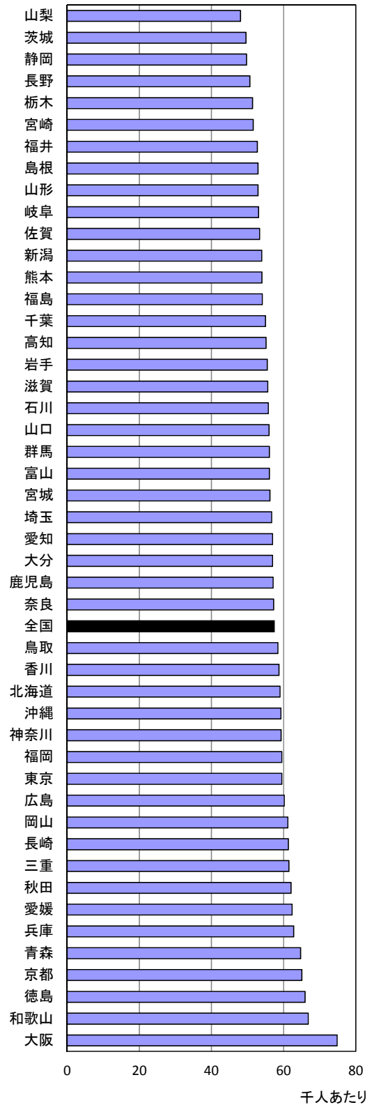
女性 平成23年 年齢調整加重障害保有割合
