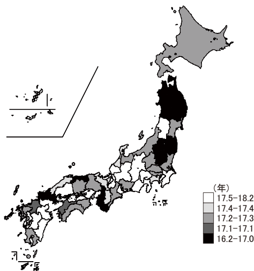
平成26年 男性 65歳 障害調整健康余命(DALE)
