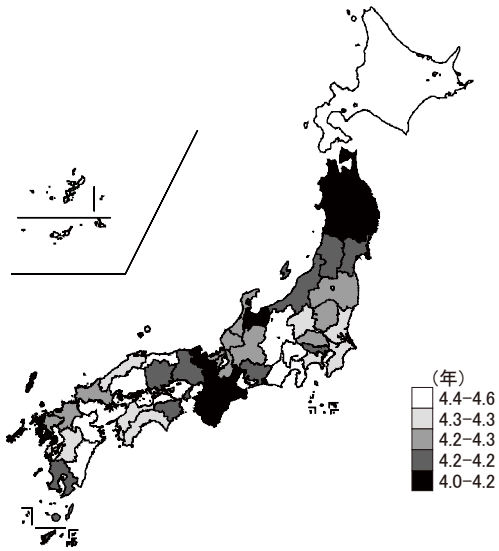
平成26年 男性 85歳 障害調整健康余命(DALE)
