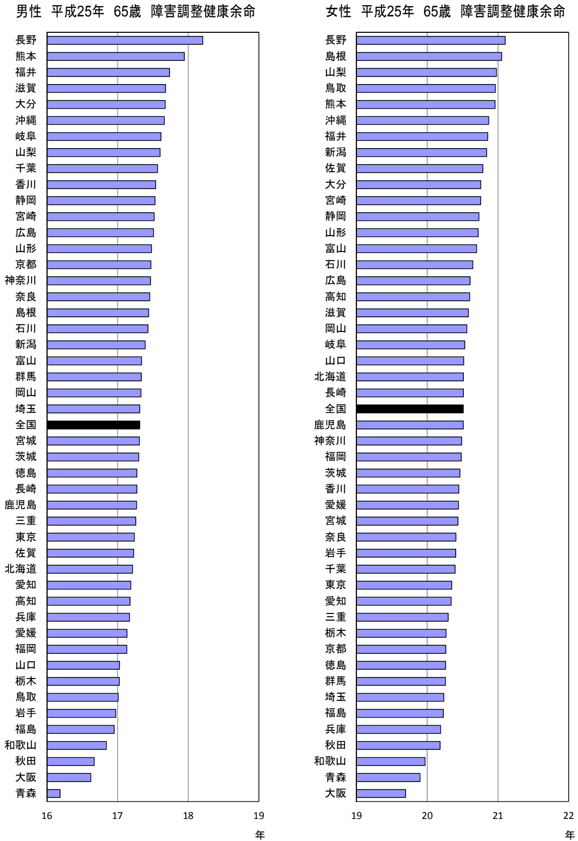
平成25年 47都道府県 65歳 障害調整健康余命(DALE)
