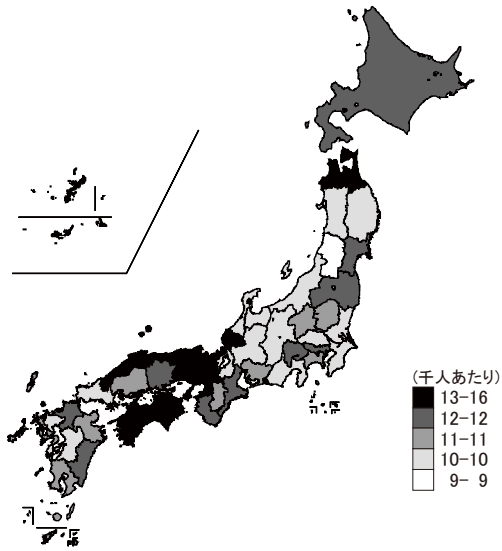
平成24年 女性 65～69歳 加重障害保有割合(WDP)
