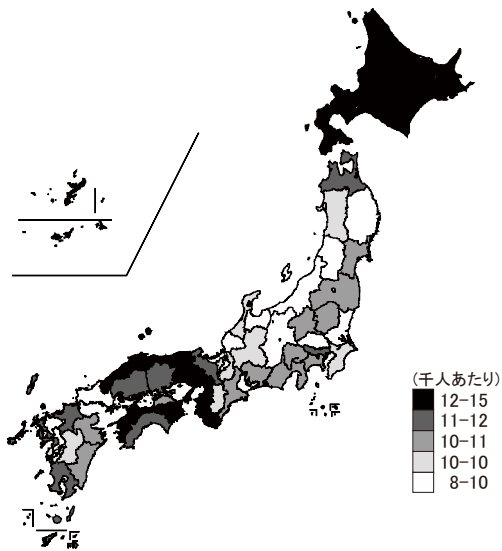
平成22年 女性 65～69歳 加重障害保有割合(WDP)
