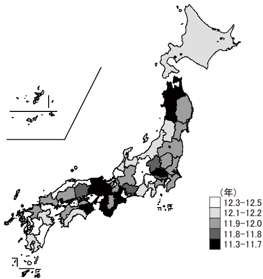
平成22年 女性 75歳 障害調整健康余命(DALE)
