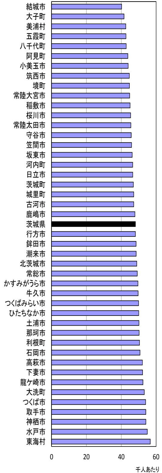
女性 平成23年 年齢調整加重障害保有割合
