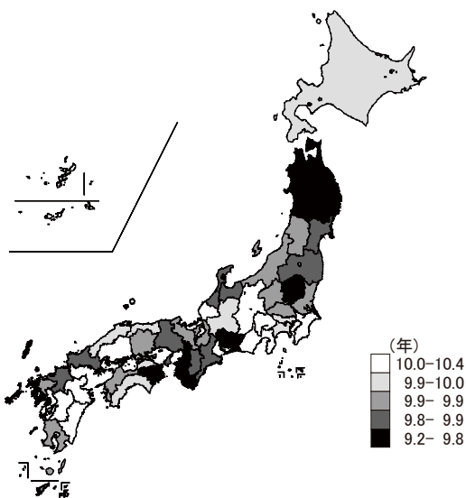
平成26年 男性 75歳 障害調整健康余命(DALE)
