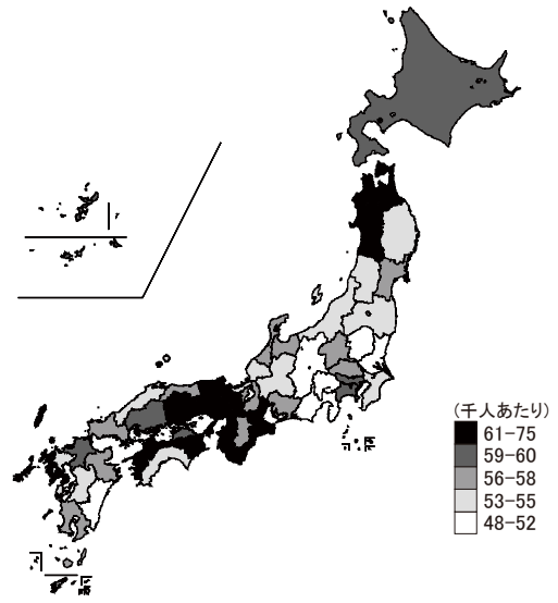
平成23年 女性 年齢調整加重障害保有割合(WDP)
