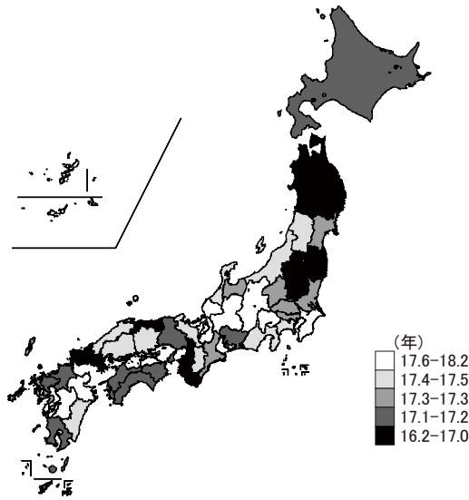
平成24年 男性 65歳 障害調整健康余命(DALE)
