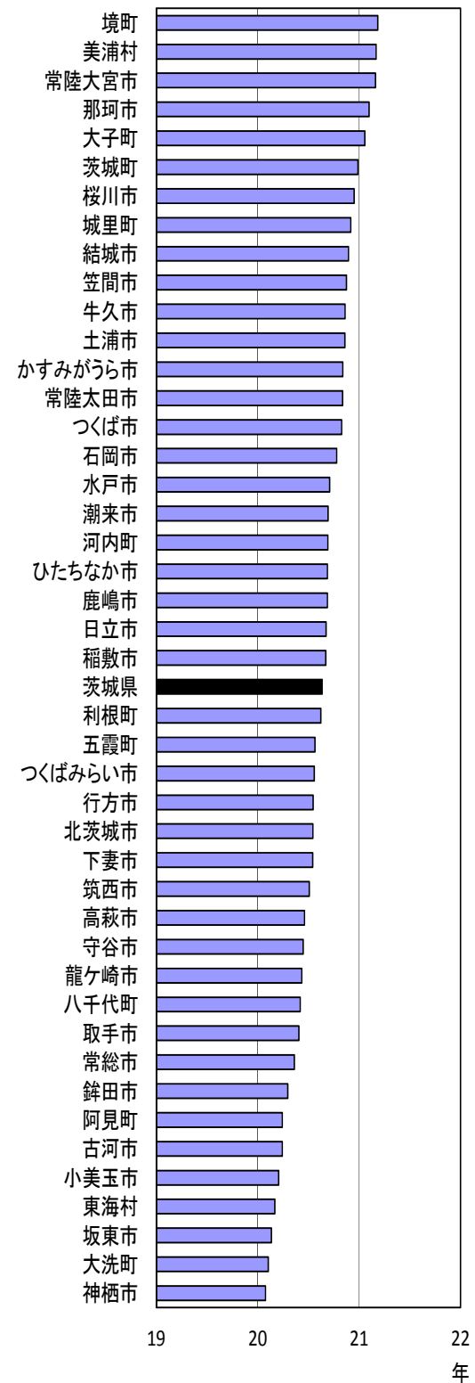
女性 平成22年 65～69歳 障害調整健康余命
