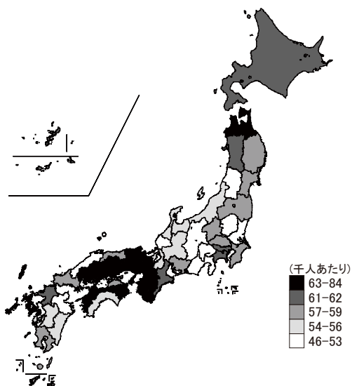
平成26年 女性 75～79歳 加重障害保有割合(WDP)
